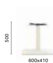
COLUMN 80x80 TOP MAX 1400x900; 1250x800 (HPL)
