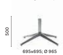
COLUMN Ø 60 TOP MAX Ø 1300
