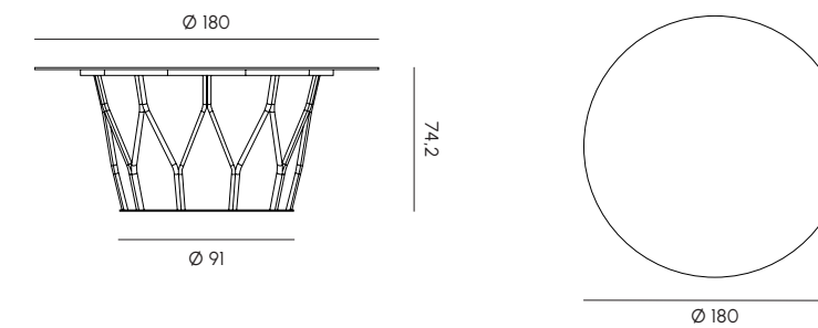
Tavolo da pranzo \varnothing 180 * Dining table \varnothing 180
