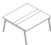
SW44 1400 / 1410 / 740 67.85 kg
