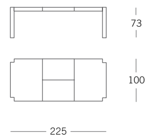
Tavolo meeting piano rivestito Upholstered meeting table Tables de réunion avec plateau revetu
