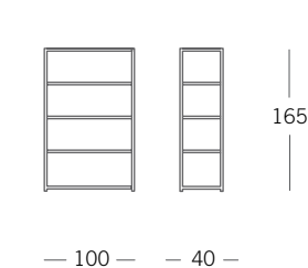
Modulo finale / centrale End / central element Elément central / Élément final
