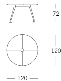
Tavoli meeting piano rivestito Upholstered meeting tables Tables de reunion avec plateau revetu
