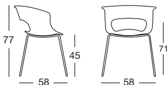
Struttura a 4 gambe 4-leg frame Art. 2690
