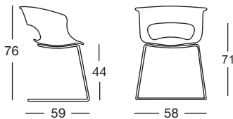
Struttura oscillante Cantilever structure Art. 2689
